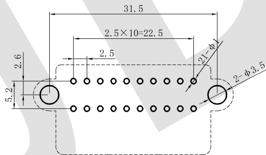
PCB板孔位示意图 公差(±0.1)
